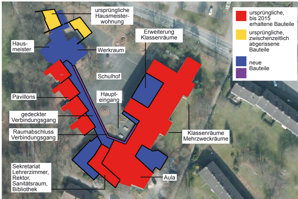
Lageplan: Adolf-Reichwein-Schule, Originalzustand und Umbauten bis zum Abriss 2015
